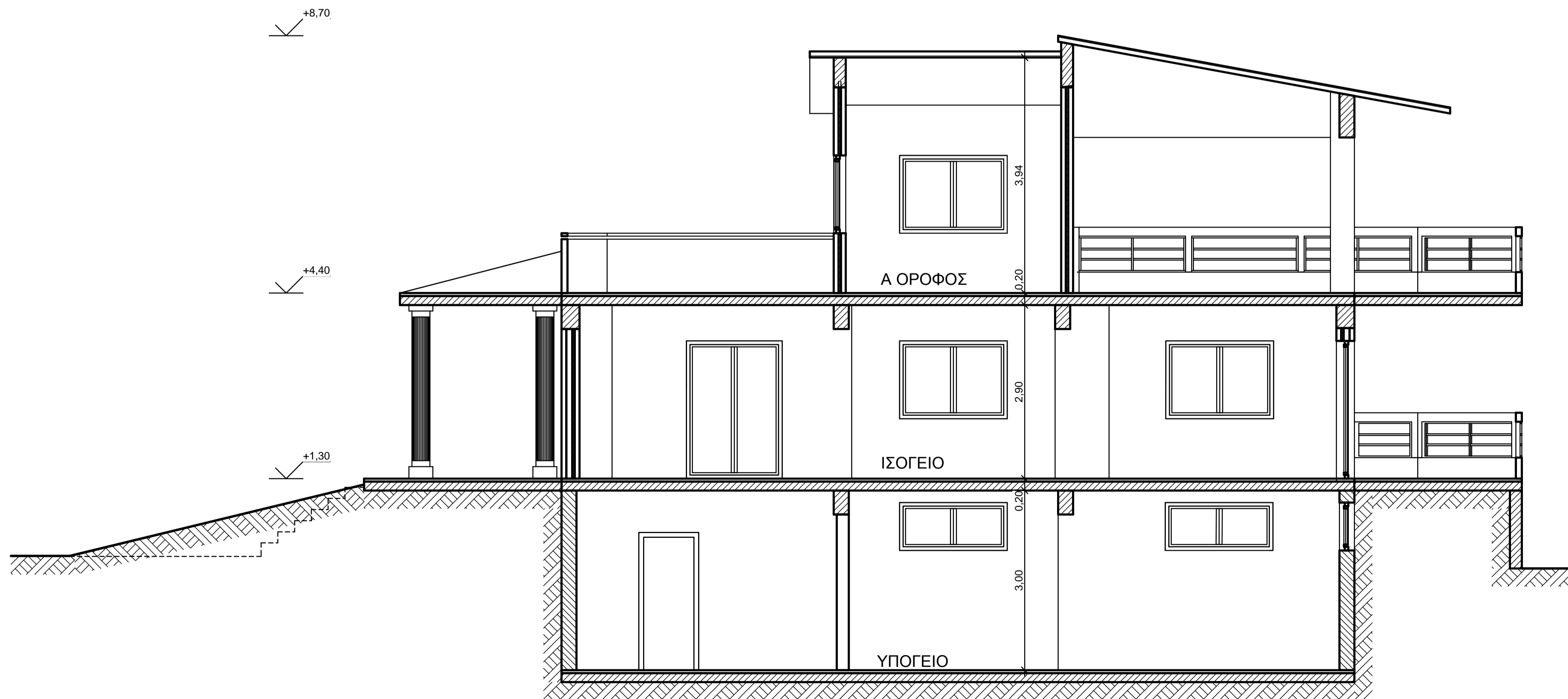
ΤΟΜΗ ΒΒ
