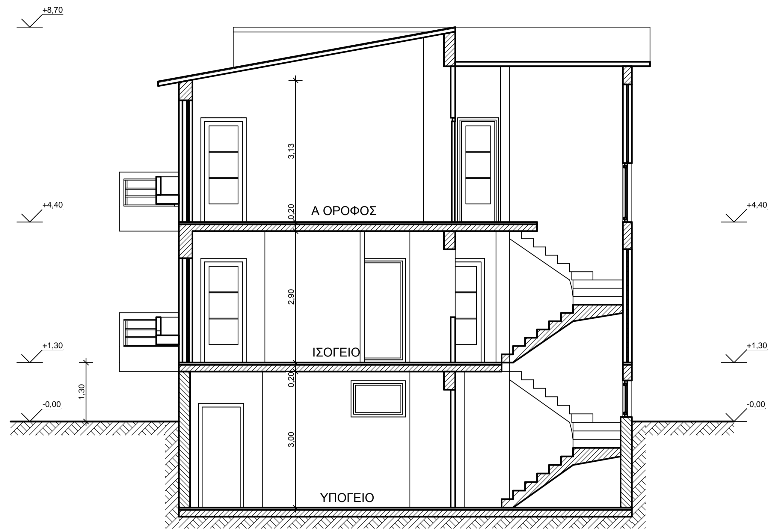
ΤΟΜΗ ΑΑ
