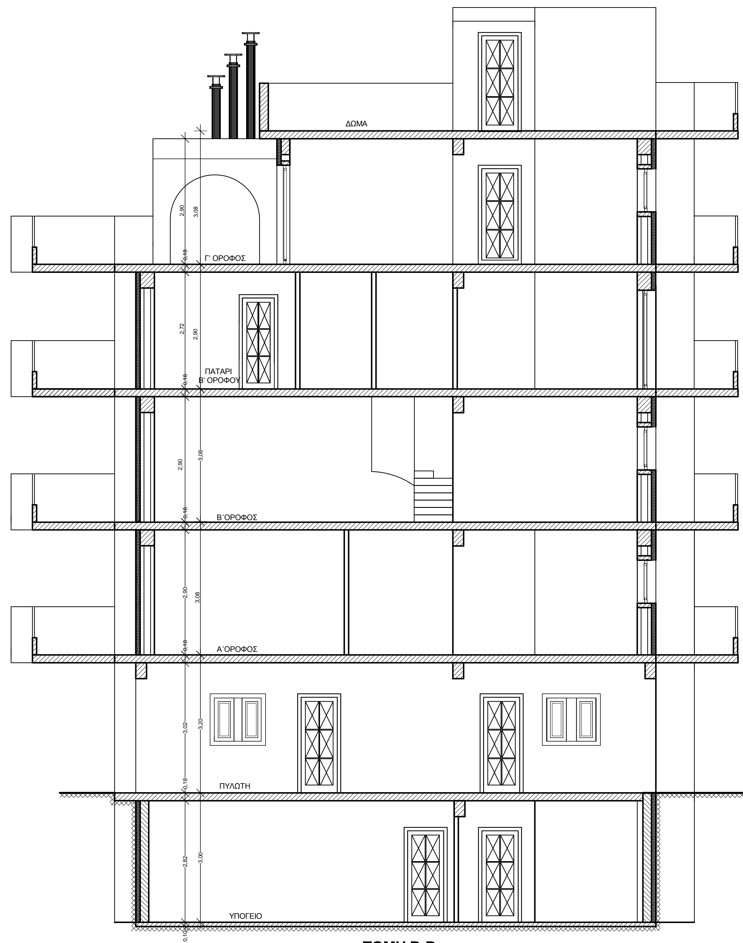
ΤΟΜΗ Β-Β
