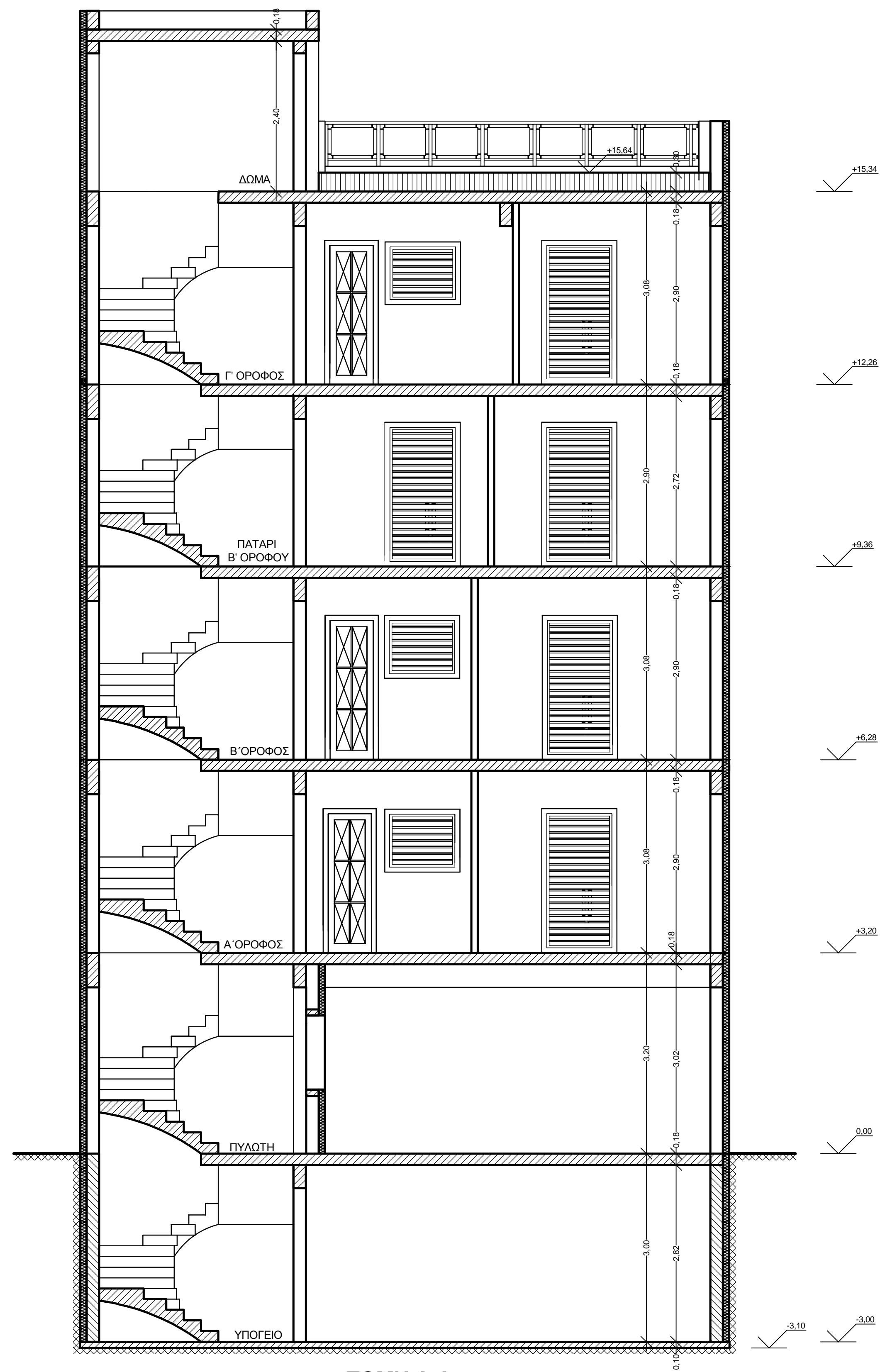
ΤΟΜΗ Α-Α
